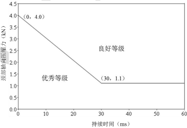
图 11 颈部压缩力 F_z 时间持续曲线
